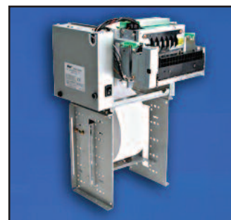
Soporte opcional para rollos de papel de 10" de diámetro
